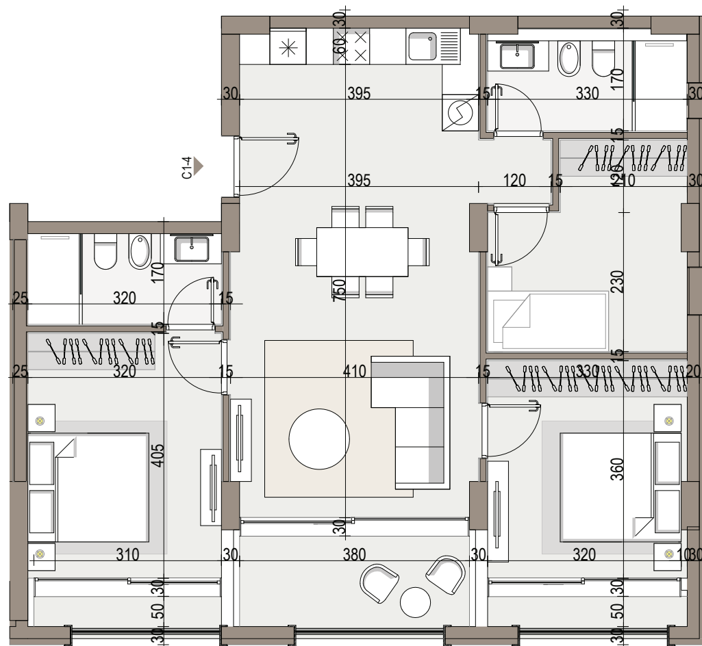
Pozicioni i apartamentit
